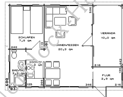
Typ D6-40+10 + Teil-Dachausbau
